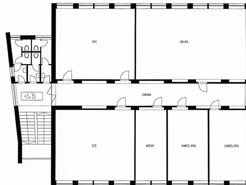
PÔDORYS 2.NP - PÔVODNÝ STAV +3.35
