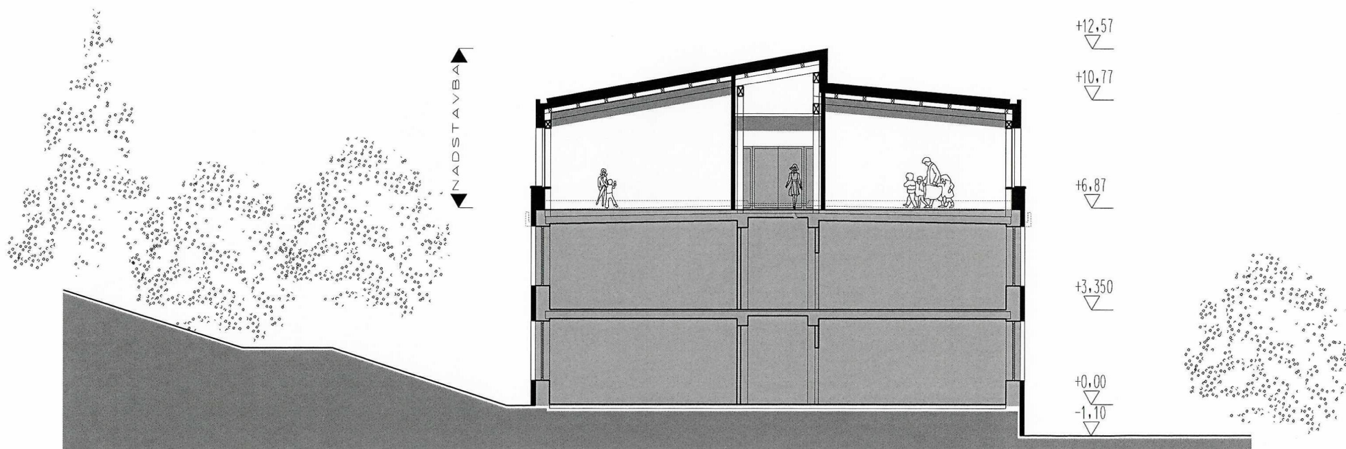
PRIEČNY REZ A-A
