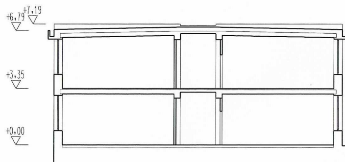
PRIEČNY REZ
