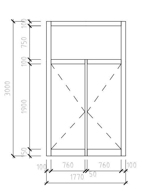
03-vstupné dvere s nadsvetlíkom 1:50
