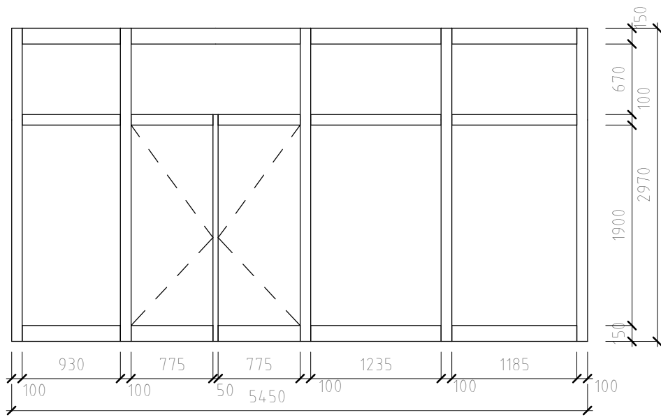
01-vstupná stena exteriér 1:50
